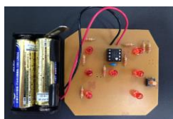
② 電子サイコロ
